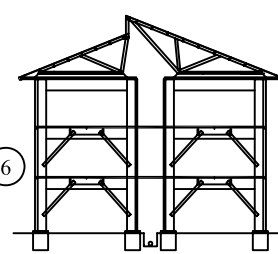
POUR UPPER FLOOR SLABS FIX TOP PRECAST LIGHTWEIGHT WALL PANELS
