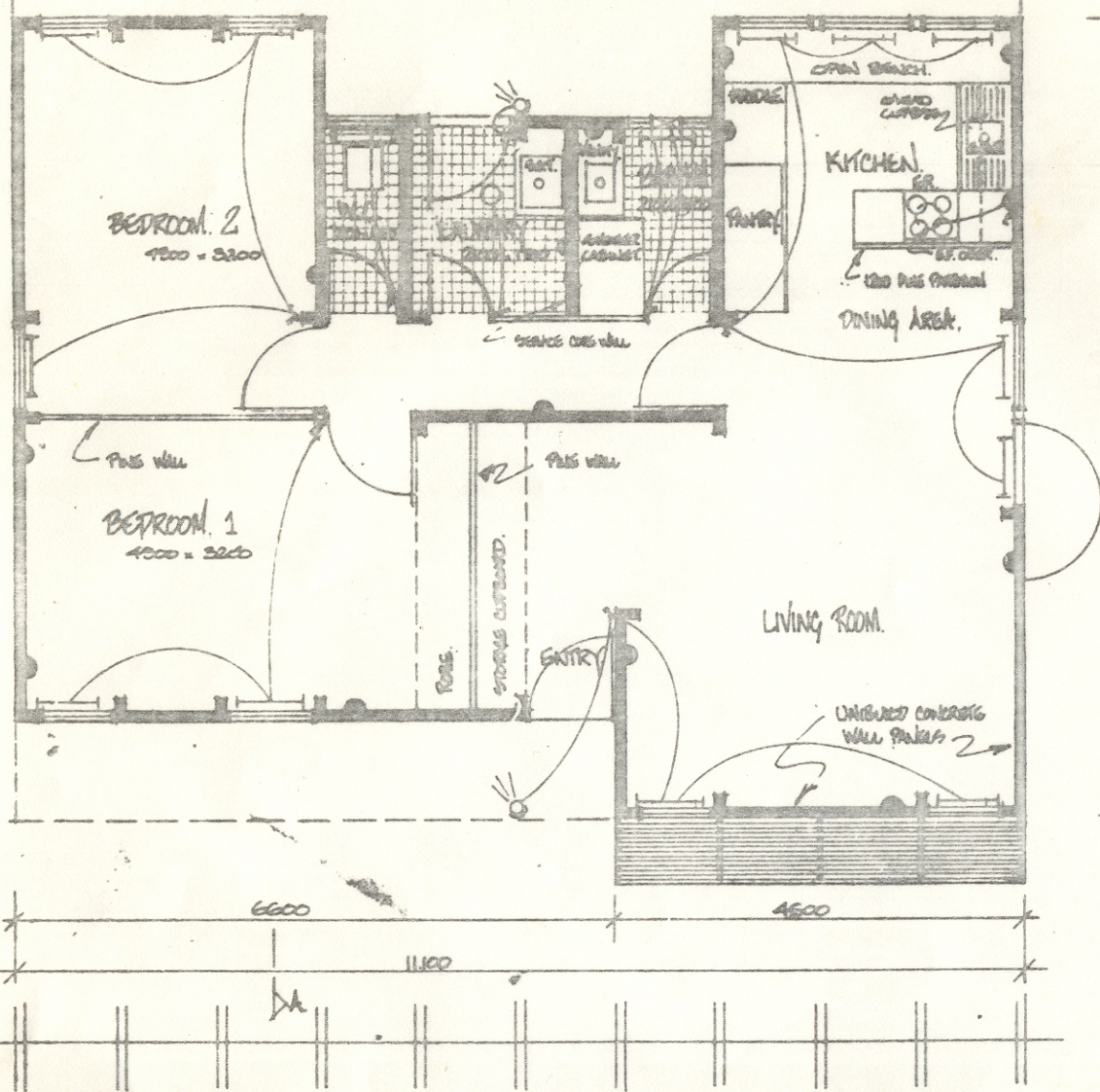
PLAN 1:50
