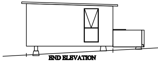
END ELEVATION
