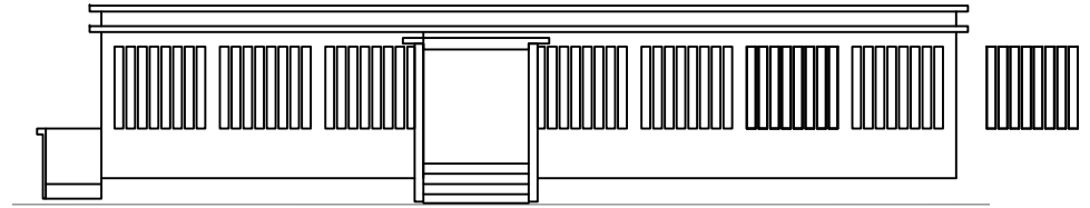
ELEVATION 4
