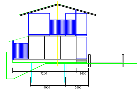
END ELEVATION
