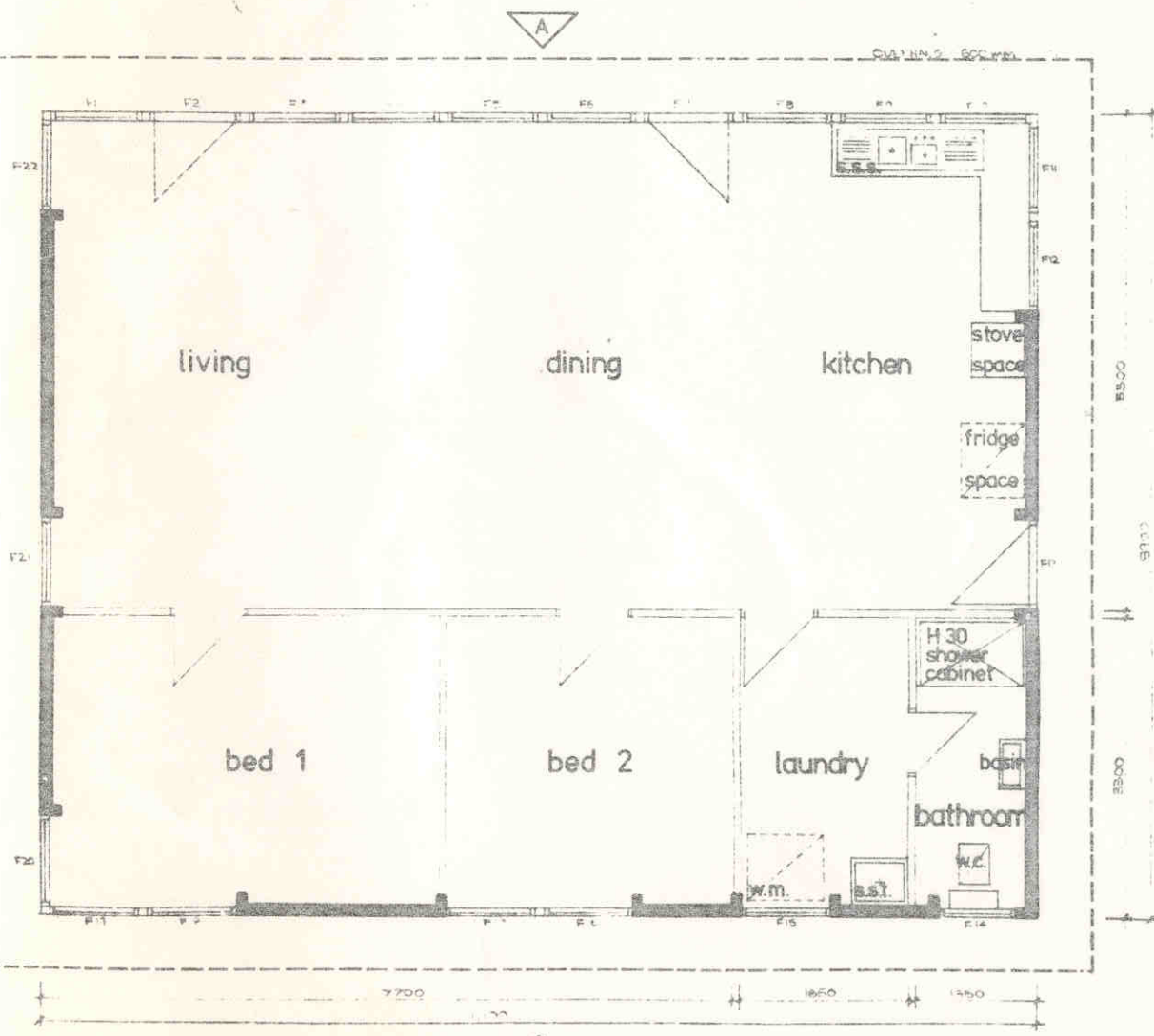
PLAN 1:50
