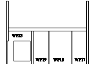
ELEVATION 4
